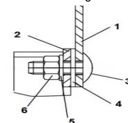
Detailzeichnung
